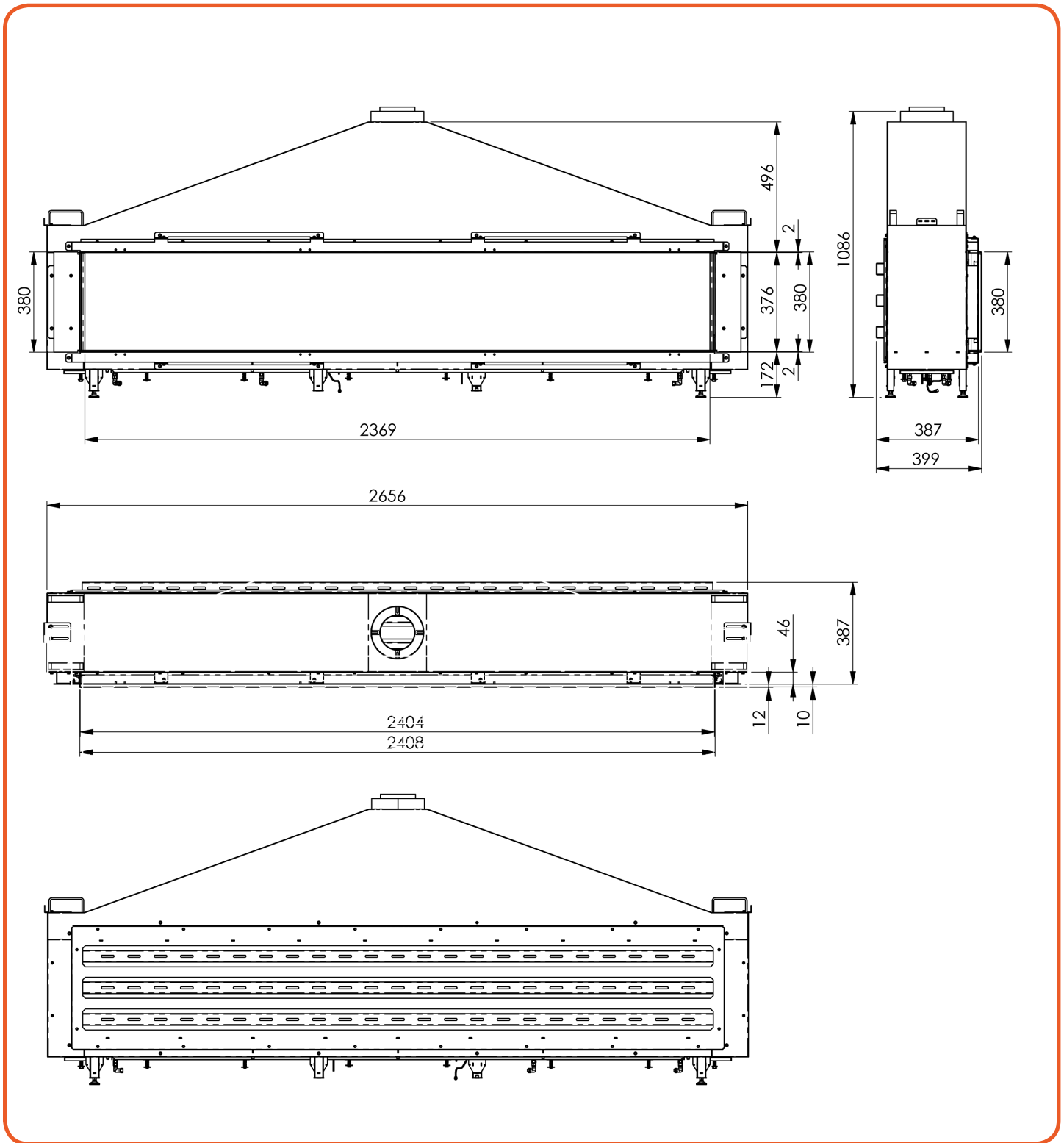
Illustration I.2 - Schéma technique du Modore 240
