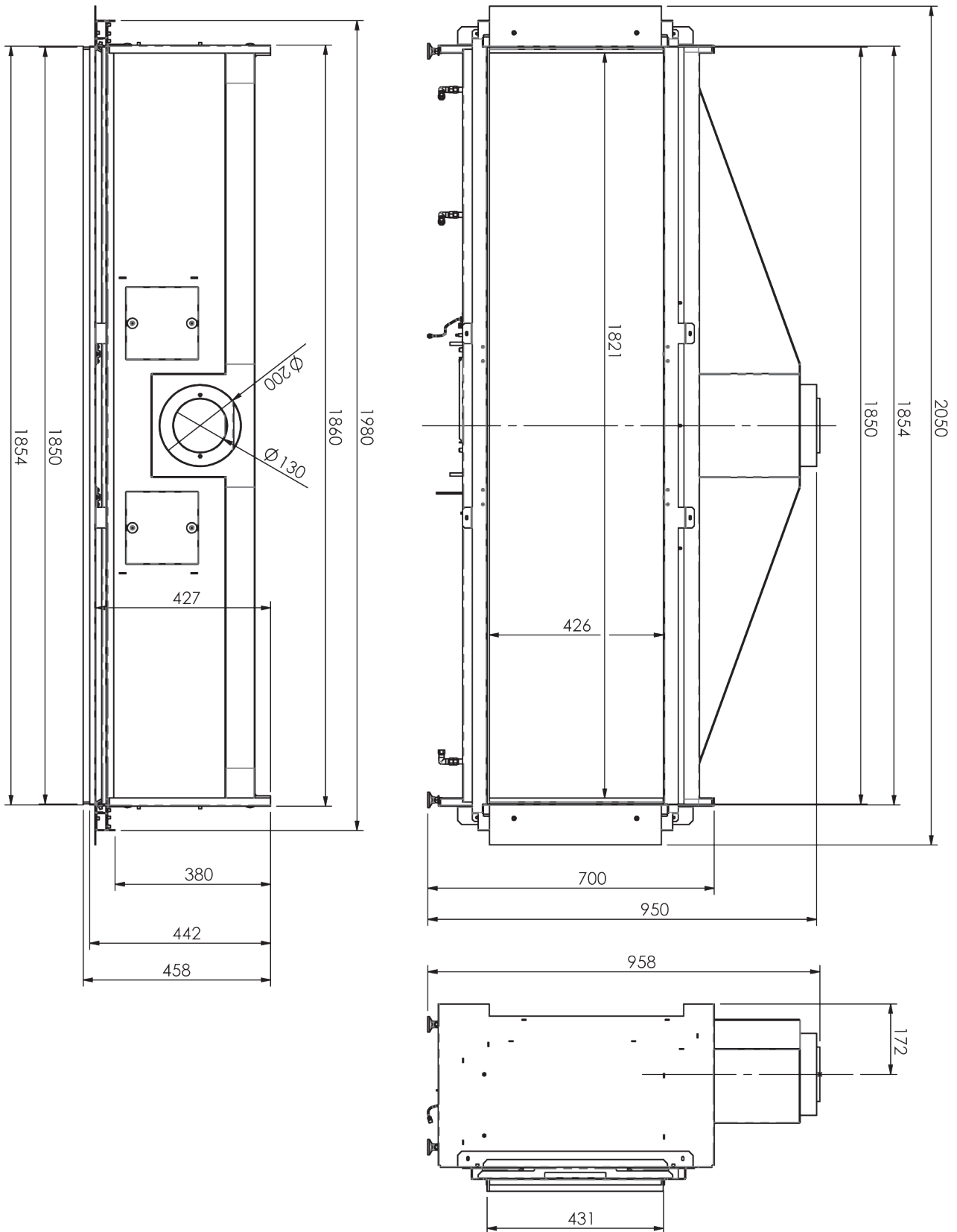
Illustration I.1 - Schéma technique du Modore 185
