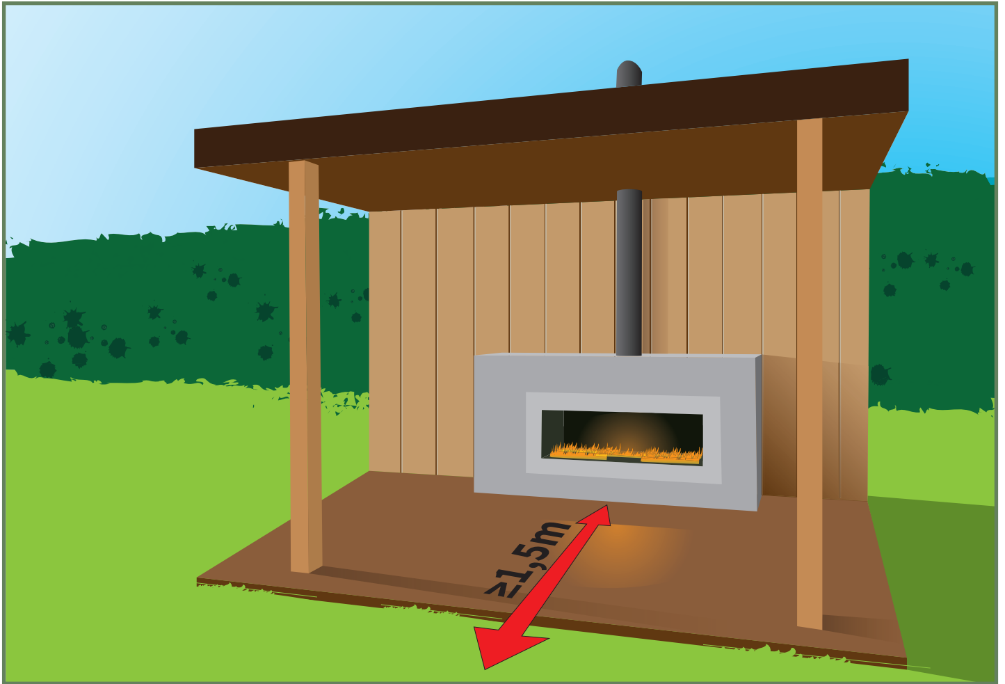
Abbildung 1 - Mindestabmessungen für Überstand bei Kaminen im Außenbereich
