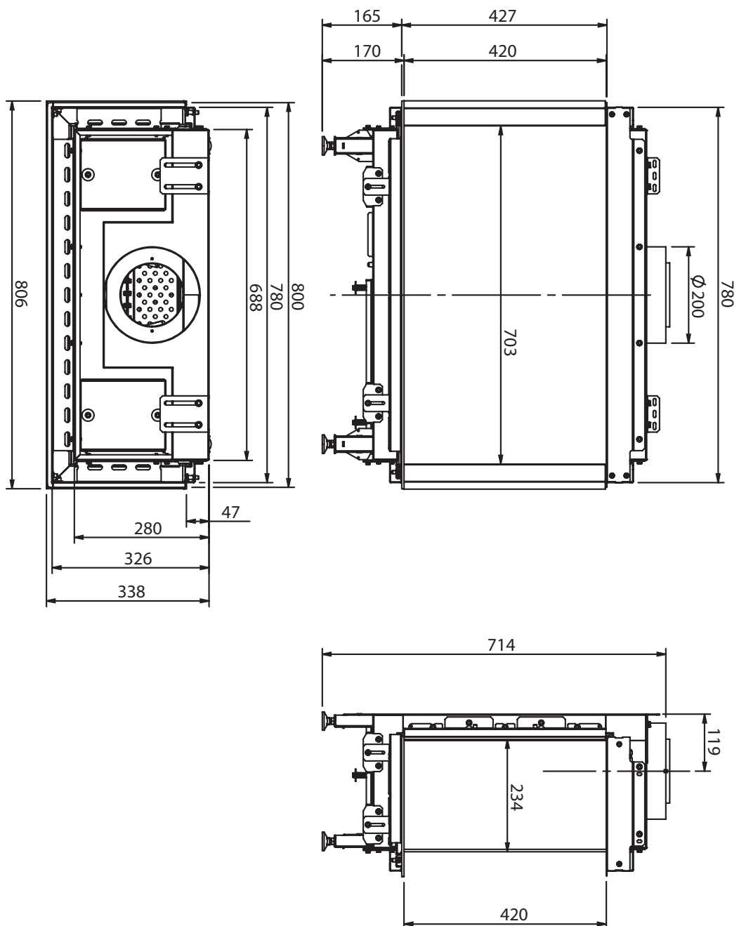
Illustration I.3 - Schéma technique du Summum 70 3S
