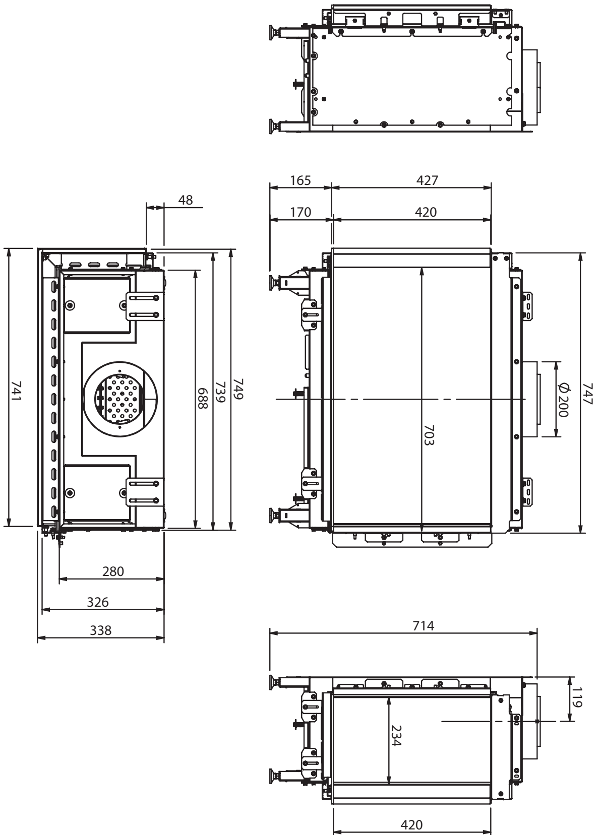
Illustration I.2 - Schéma technique du Summum 70 C
