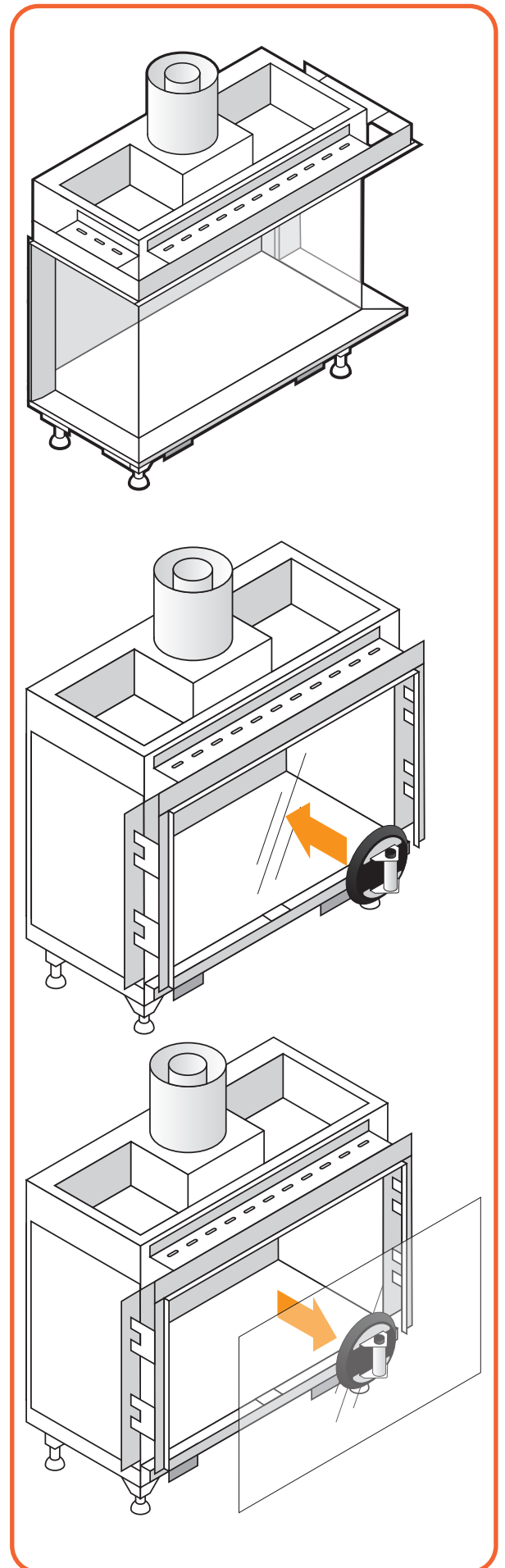
Ill. 10.1 - Exemple du Summum 70
